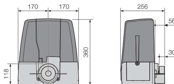
SLX3024CB
