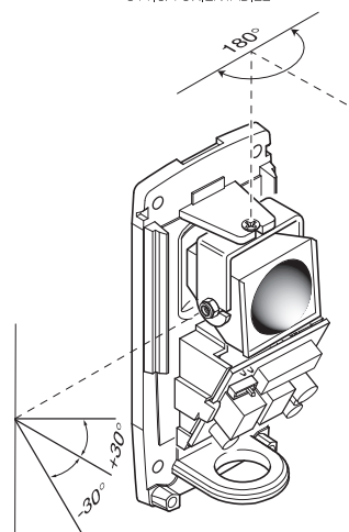
OTTICA ORIENTABILE
