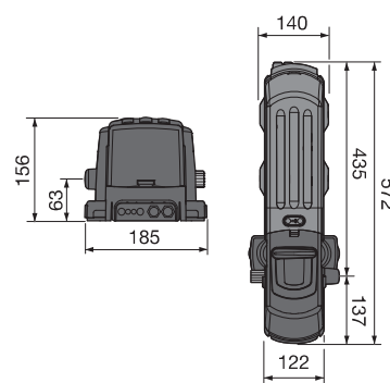
GLB249M - GLB248M
