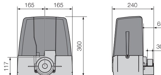
SLX824CB - SLX1524CB
