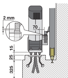
SL524 SL524CB
