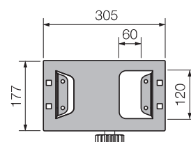
BASE DI FISSAGGIO CODICE DI RICAMBIO RPIAFAVOZ
