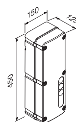
CC242EFAMCB
