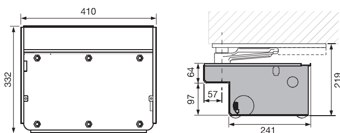
HL MOLE24 - HL MOLE230
