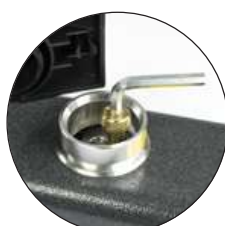
SBLOCCO - BLOCCO A CHIAVE ESAGONALE
