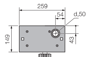
BASE DI FISSAGGIO CODICE DI RICAMBIO PIAFACE300AS
