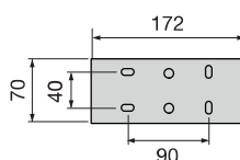
BASE DI FISSAGGIO CODICE DI RICAMBIO 999750
