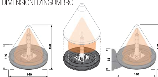
APPLICAZIONE A COLONNA
