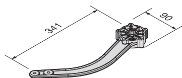
DIMENSIONI BRACCIO DRITTO BL TEN2
