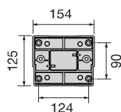
BASE DI FISSAGGIO CODICE DI RICAMBIO 999533
