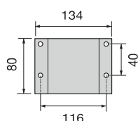
BASE DI FISSAGGIO CODICE DI RICAMBIO 999626
