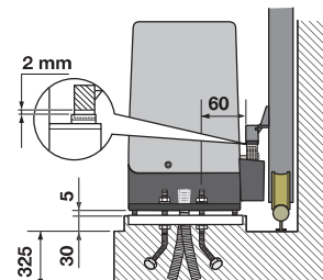
SL EVO 2000
