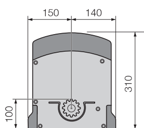
SL524 - SL524CB
