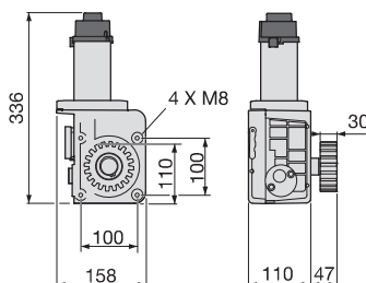
SLi724
