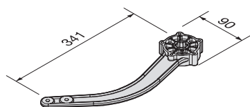
DIMENSIONI BRACCIO DRITTO BL TEN1
